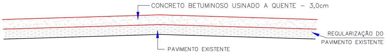
DET. DOS REVESTIMENTOS CBUQ S/ESC.
