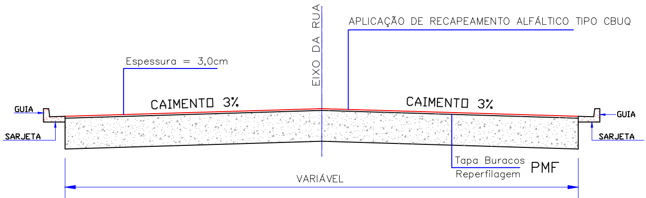
PERFIL TRANSVERSAL DA RUA S/ESC.
