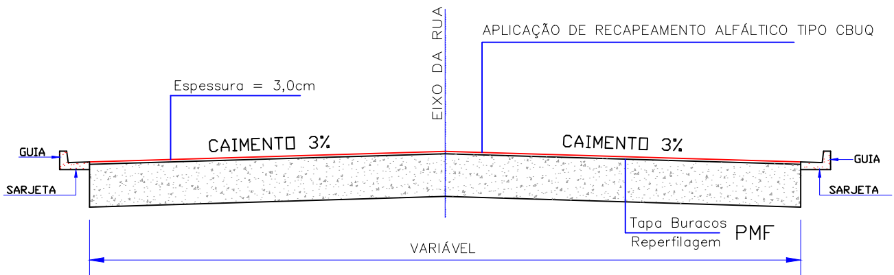
PERFIL TRANSVERSAL DA RUA S/ESC.
