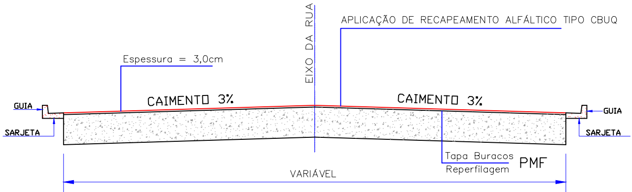
PERFIL TRANSVERSAL DA RUA S/ESC.
